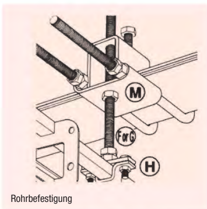
Rohrbefestigung
