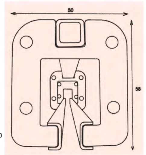
Kompaktschiene C-400 (Originalgröße) Alle Angaben in mm
